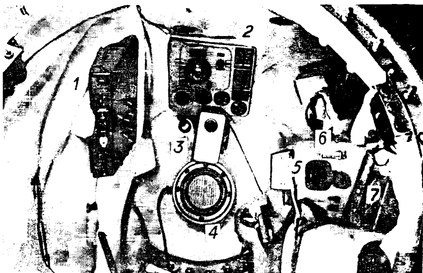
Avaruuslentäjän hytin sisäkuva avaruusaluksessa Vostok 1 — lentäjän ohjaimet; 2 — kojetaulu karttapalloonine; 3 — televisiokamera; 4 — ikkuna, jossa on optinen suunnasluksilaitte; 5 — aluksen suunnasluksilaitteen ohjain; 6 — radiovastaanotin; 7 — ravintosäiliö.
