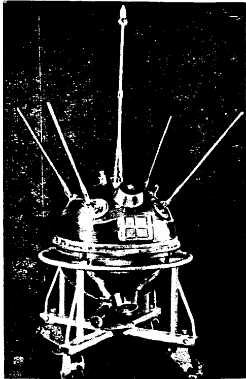
Neuvostolaisen avaruusraketin, aurion keinotekoisien seuralaisen, tulkimuskojeistojen kammio.
