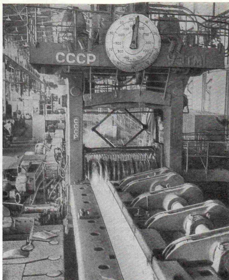
Intia. Neuvostoliiton avustamana rakennettu ja neuvostoliittolaisella kalustuksella varustettu Bhilain terästehdas
