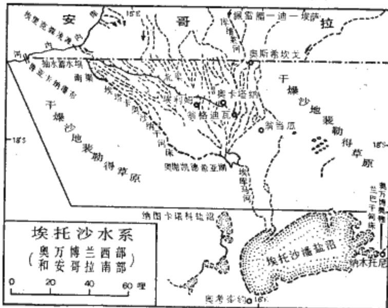
图 5 埃托沙水系和埃托沙潘盐沼
