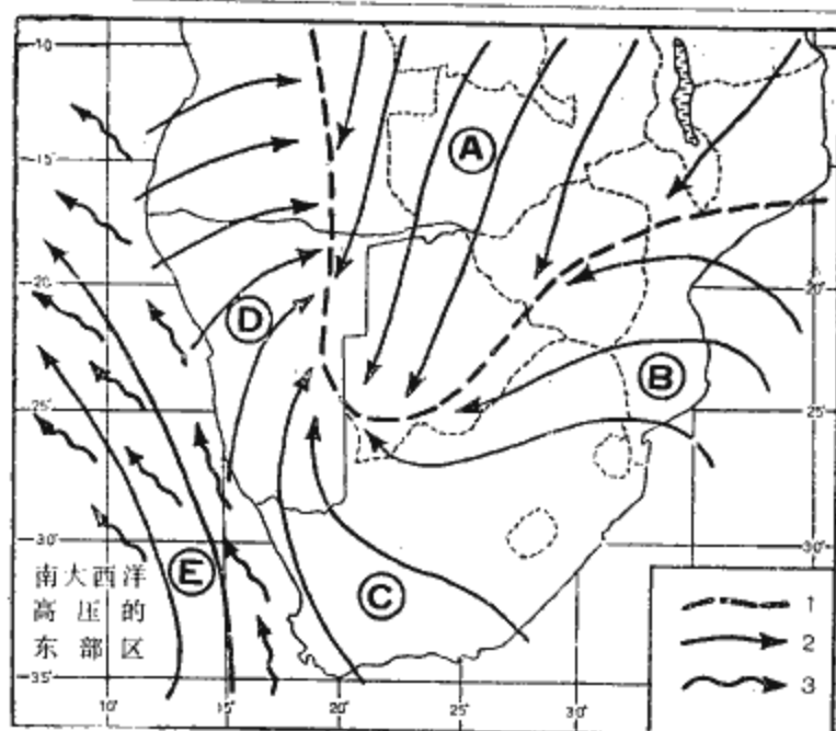
图 6 西南非洲气候因素 夏季主要的气流和洋流
